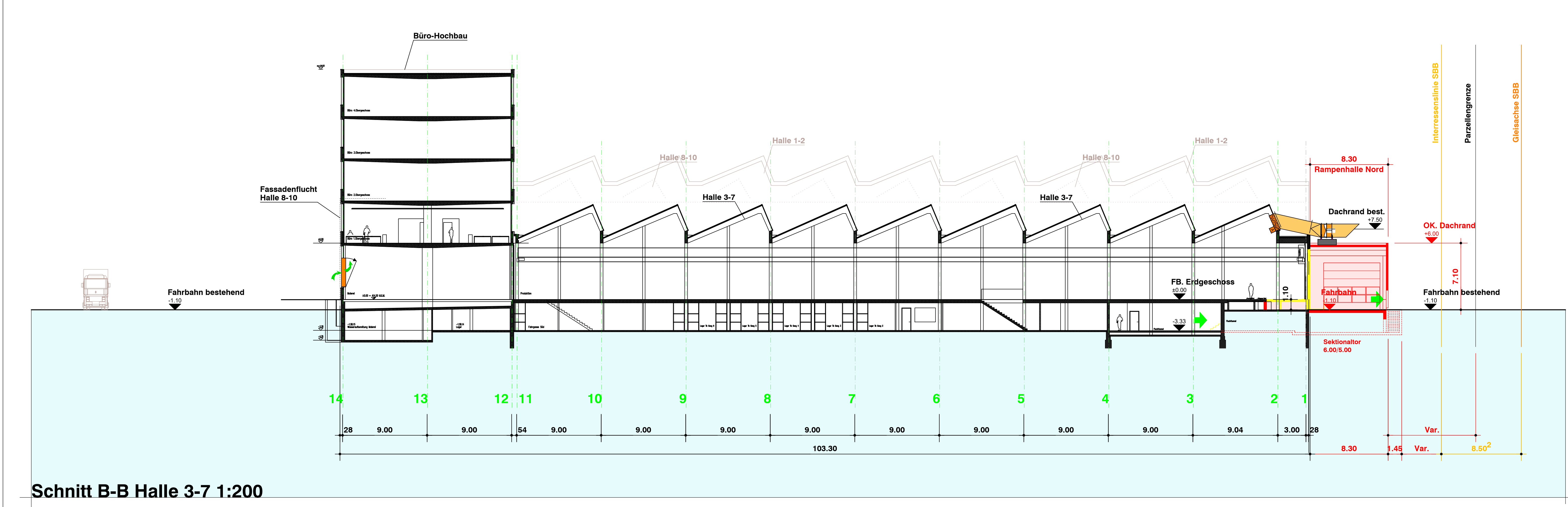
Schnitt B-B Halle 3-7 1:200
