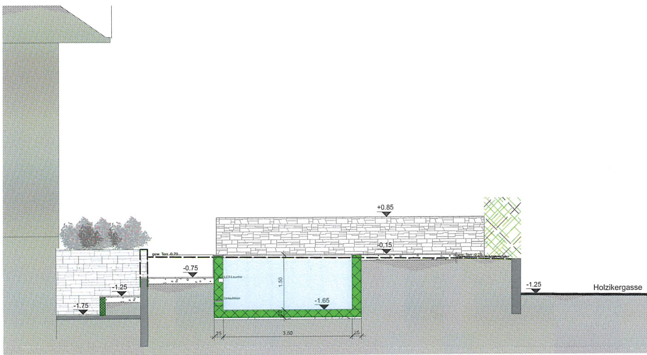
Schnitt E-E
