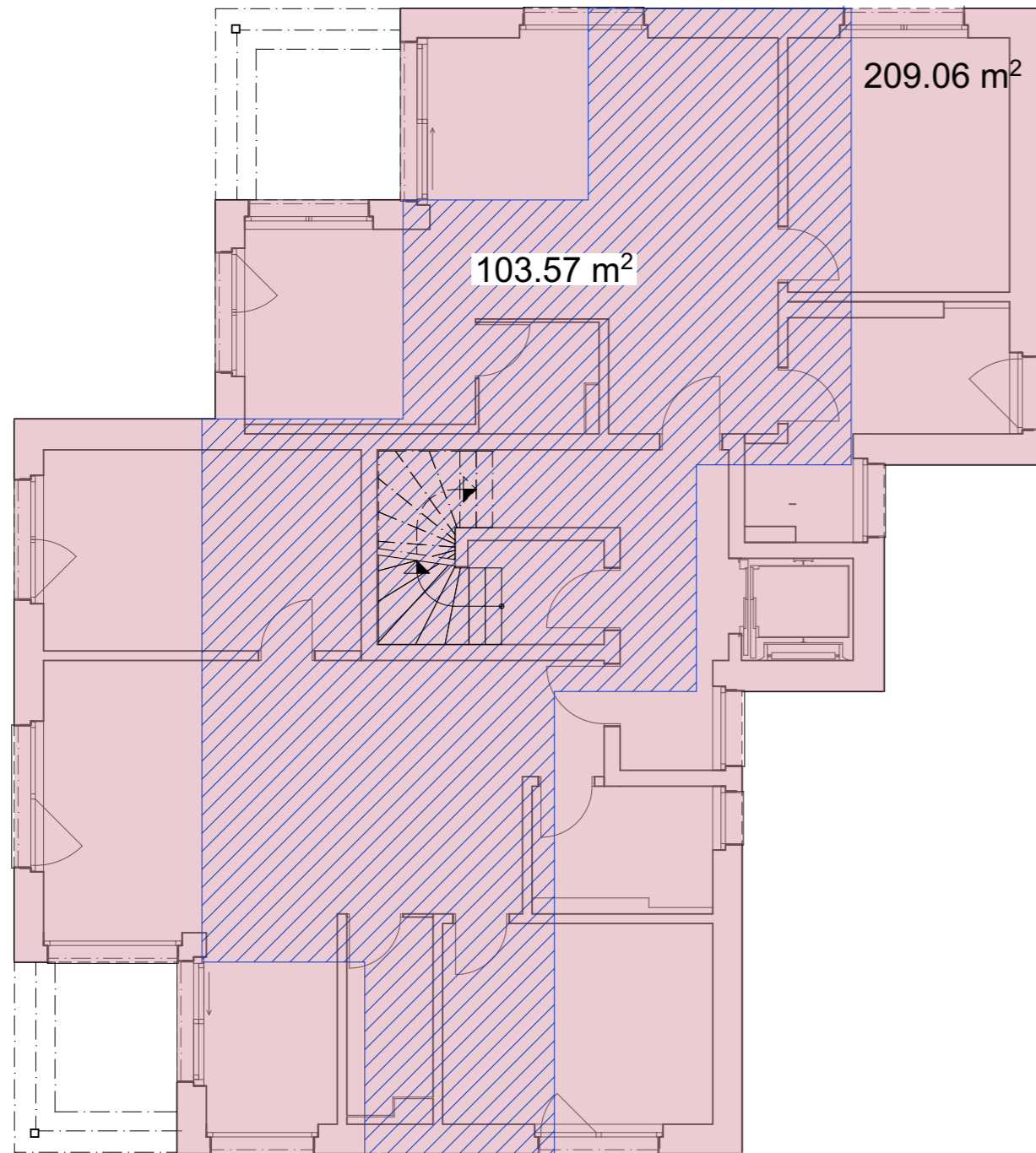
3. OBERGESCHOSS 1:100
