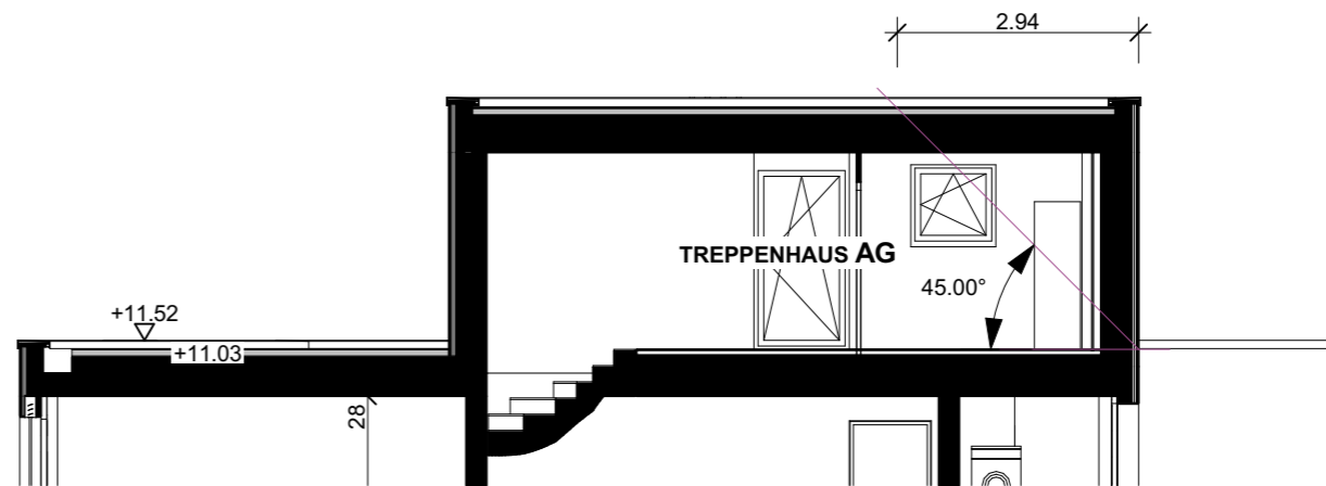
SCHNITT 1 1:100
