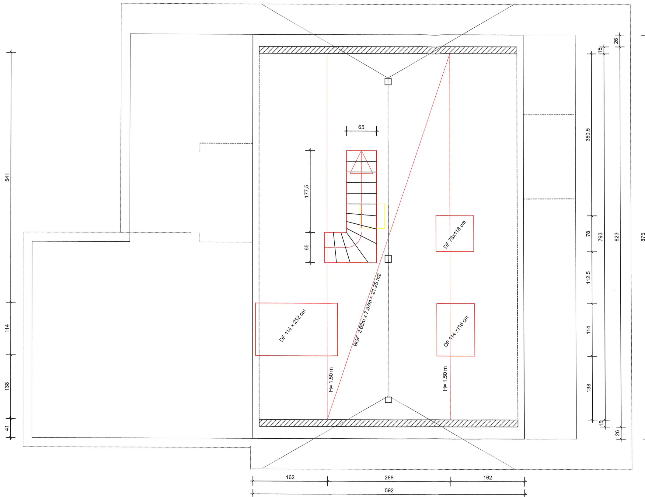
Grundriss Dachgeschoss
