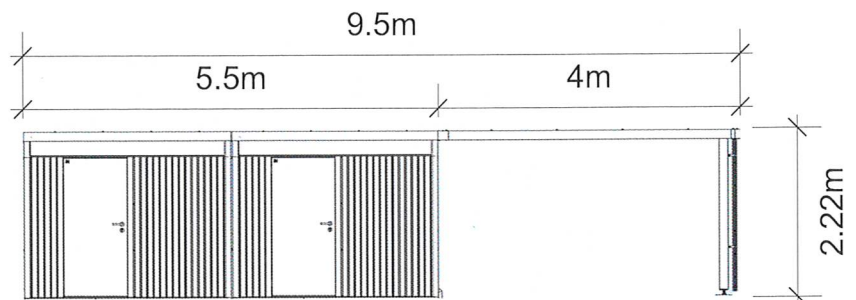
Ansicht Südost
