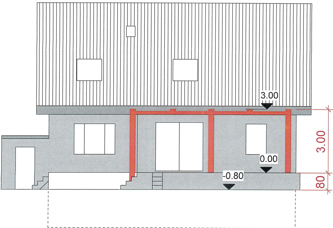
SÜDFASSADE
