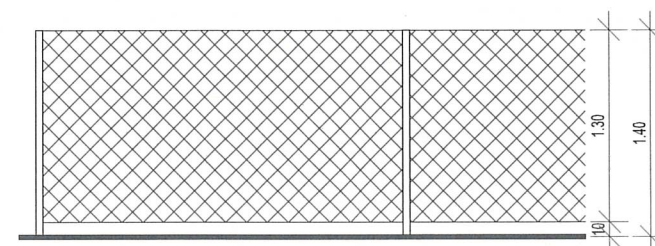
Ansicht Zaun
